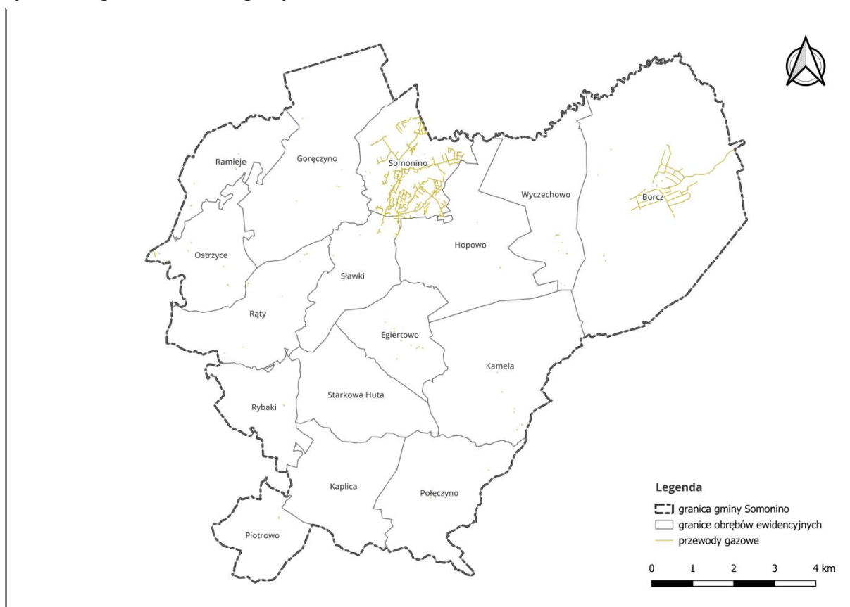
Ryc. 38. Sieć gazowa na terenie gminy Somonino
