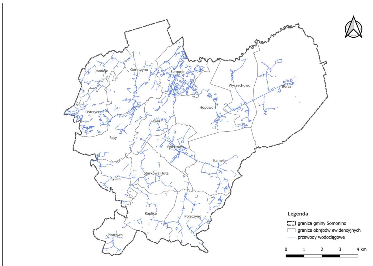
Ryc. 37. Sieć wodociągowa na terenie gminy Somonino
