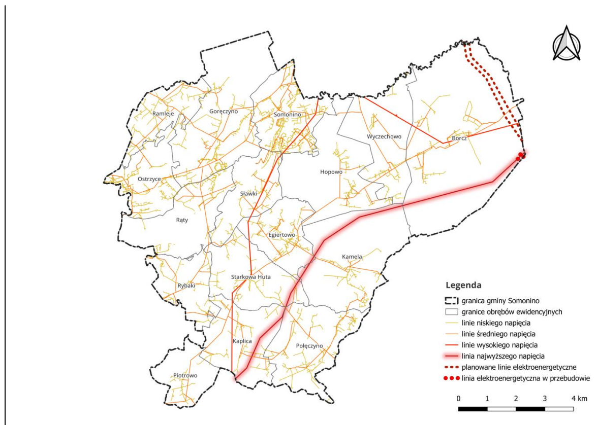
Ryc. 40. Sieć elektroenergetyczna na terenie gminy Somonino
