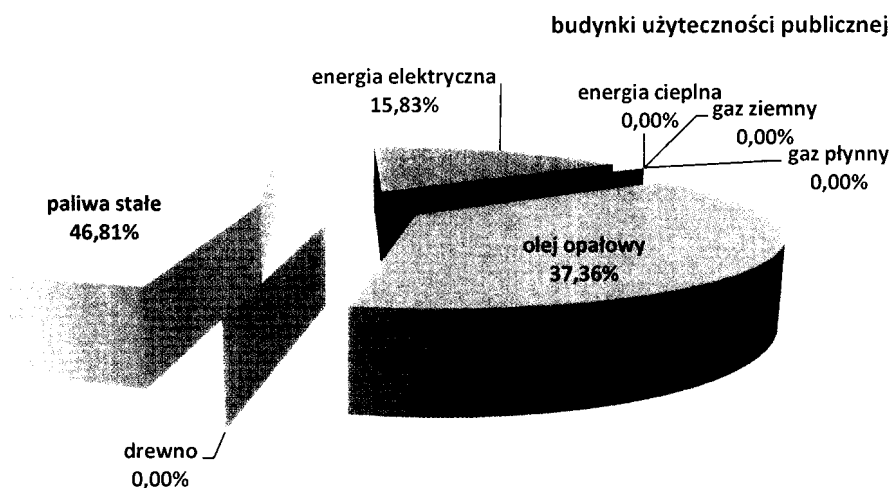
Rysunek 14. Struktura emisji CO 2 wynikającej ze zużycia energii elektrycznej, cieplnej oraz poszczególnych paliw w sektorze budynków użyteczności publicznej 27
