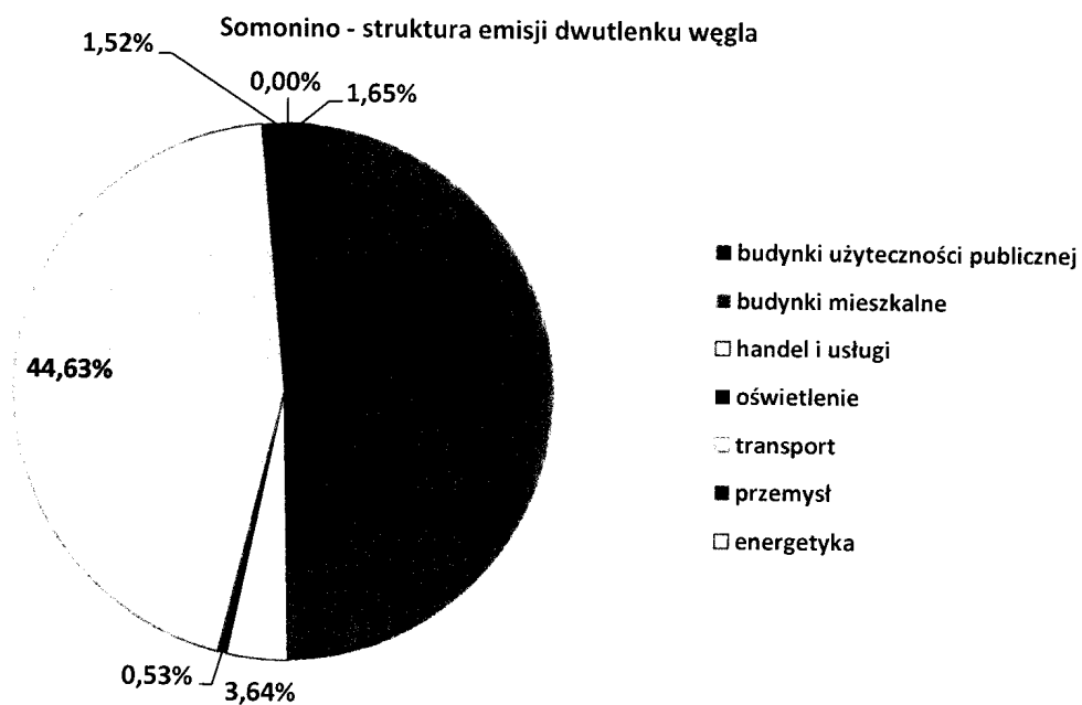
Rysunek 6. Struktura emisji ekwiwalentnego dwutlenku węgla w Gminie Somonino 13
