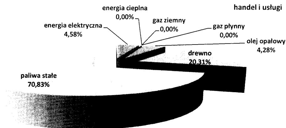
Rysunek 13. Struktura emisji CO 2 wynikającej ze zużycia energii elektrycznej, cieplnej oraz poszczególnych paliw w sektorze handlu i usług 26
