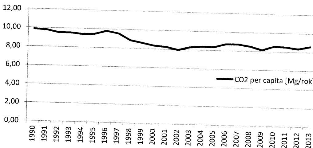
Rysunek 17. Wskaźnik emisji CO 2 per capita [Mg/rok] (źródło: opracowanie własne na podstawie danych GUS, KOBIZE)
