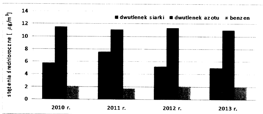
Rysunek 2. Stężenia średnioroczne dwutlenku siarki, dwutlenku azotu i benzen w rejonie gminy Somonino w latach 2010-2013 (Źródło: Roczna ocena jakości powietrza w województwie pomorskim. Raport za rok 2013 r. WIOŚ w Gdańsku)
