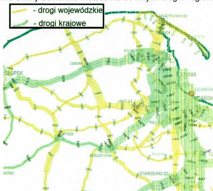
Ryc. 5. Średni dobowy ruch pojazdów na drogach krajowych i wojewódzkich centralnej części województwa pomorskiego wg GPR 2015
