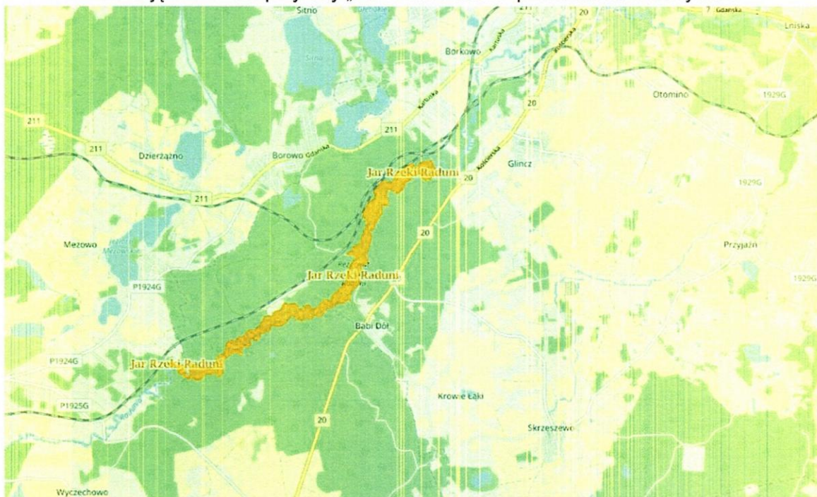
Ryc. 29. Lokalizacja rezerwatu przyrody „Jar Rzeki Raduni”
