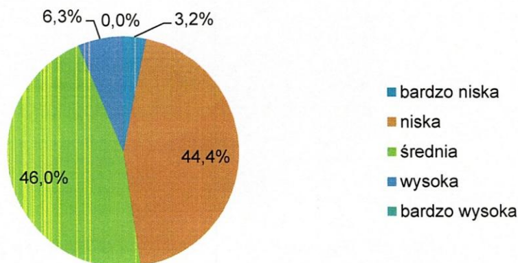
Ryc. 18. Zasobność w potas gleb z terenu Gminy Somonino
