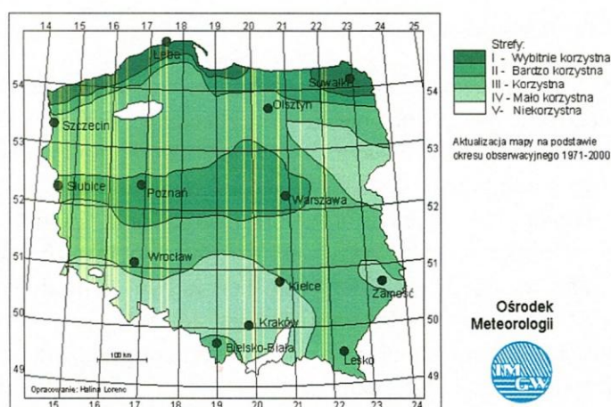
Ryc. 2. Strefy energetyczne wiatru w Polsce
