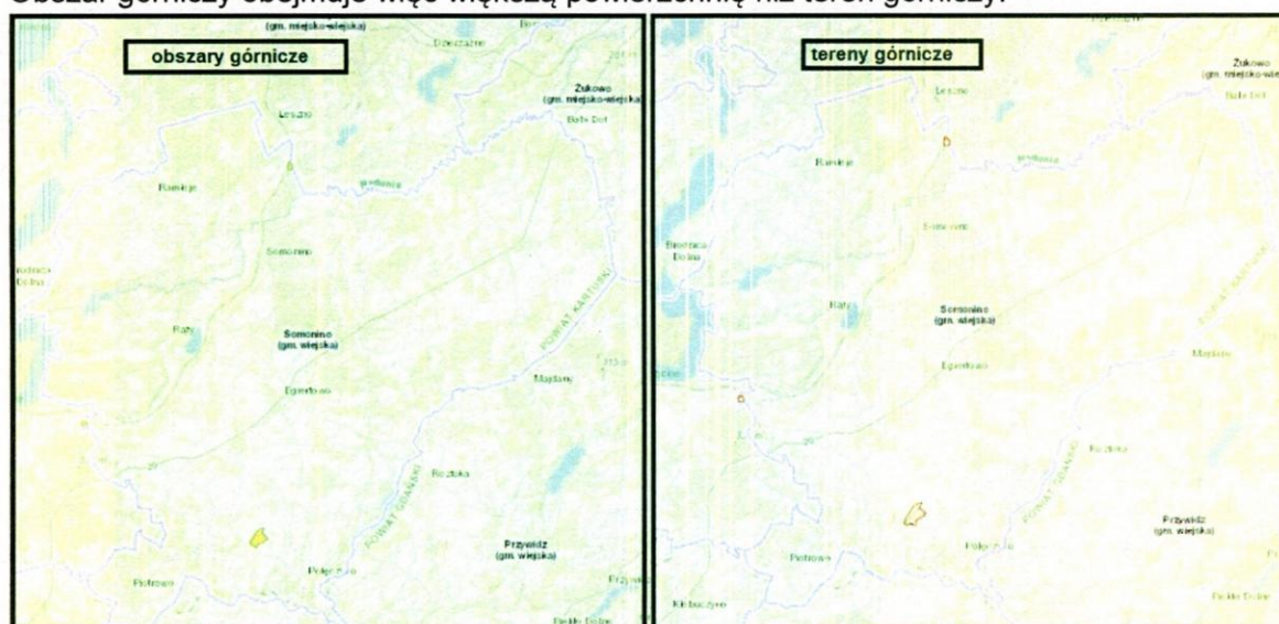
Ryc. 11. Granice obszarów górniczych i terenów górniczych w Gminie Somonino Źródło: dane Państwowego Instytutu Geologicznego
