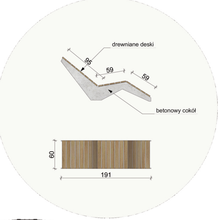
LEŻAK 1:50
