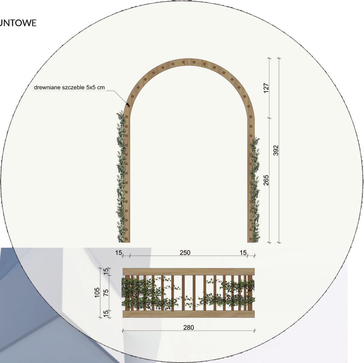
PERGOLA 1:50
