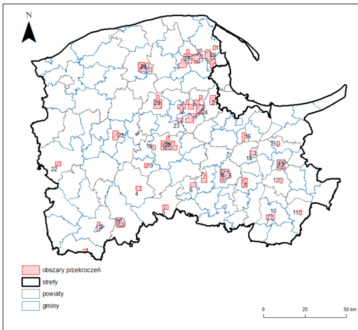
Ryc. 14. Zasięg podobszarów przekroczeń poziomu docelowego benzo(a)pirenu w pyłe zawieszonym PM10 w województwie pomorskim w 2021 roku
