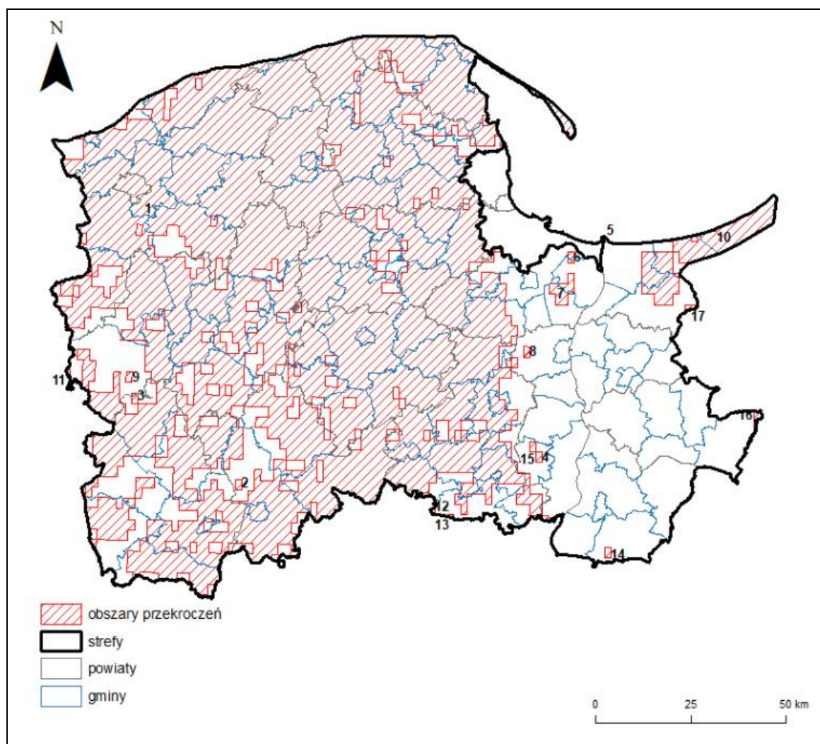
Ryc. 16. Zasięg podobszarów przekroczeń poziomu celu długoterminowego ozonu ustanowionego ze względu na ochronę roślin w województwie pomorskim w 2021 roku
