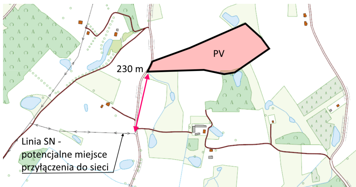
Rys. 7 Linia SN - potencjalne miejsce przyłączenia
