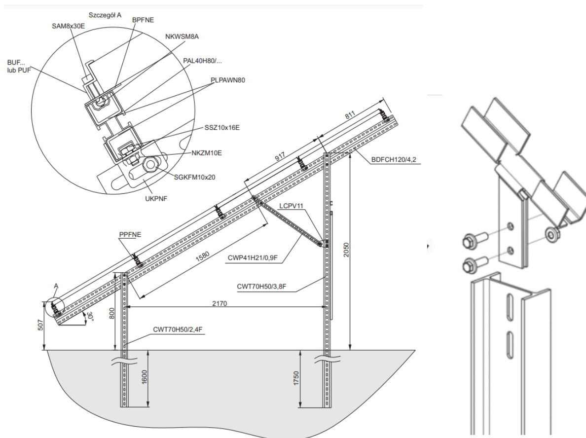
Zdj. 16 System montażu konstrukcji wsporczej
