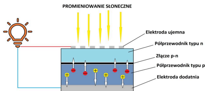
Rys. 4 Zjawisko fotowoltaiczne
